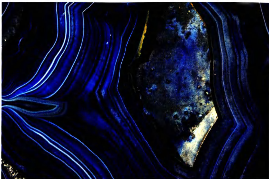
Агат
