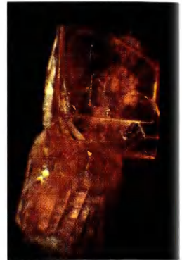
Лантанит
