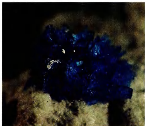
Пентагонит
