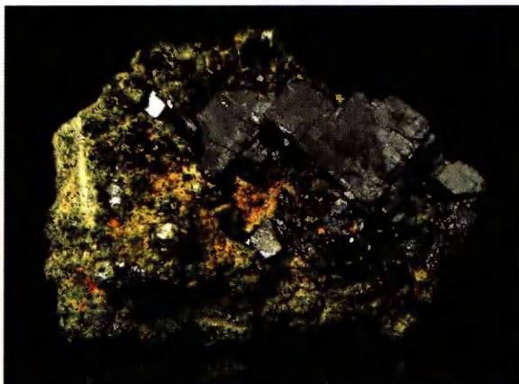
Перовскит
