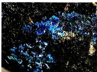
Самплеит
