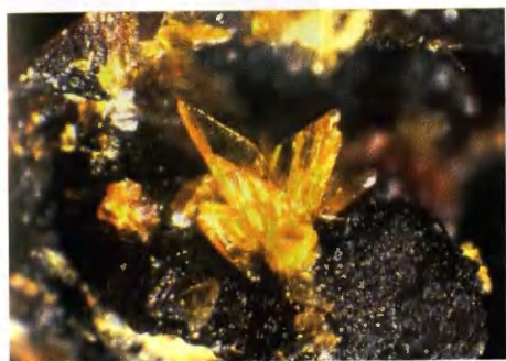
Стюартит
